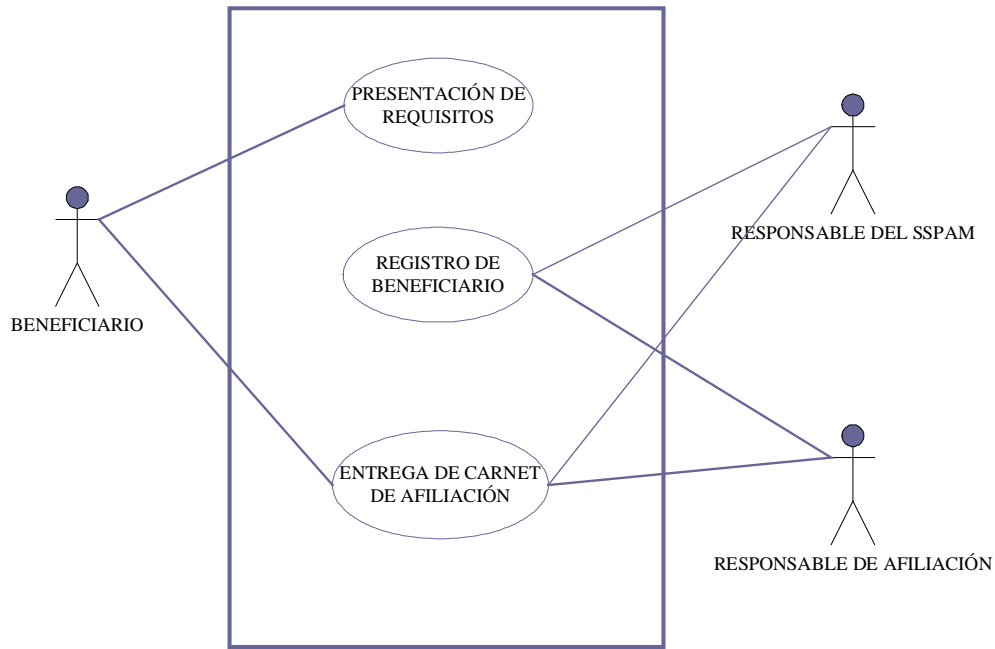
Figura 3.4 Caso de Uso: Inscripción Fuente: Elaboración Propia
