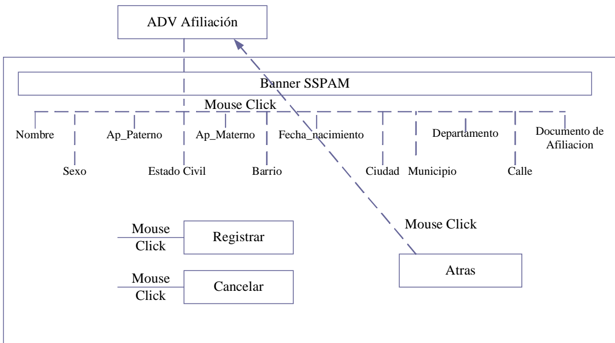
Figura 3.22 ADV Afilación Fuente: Elaboración Propia
