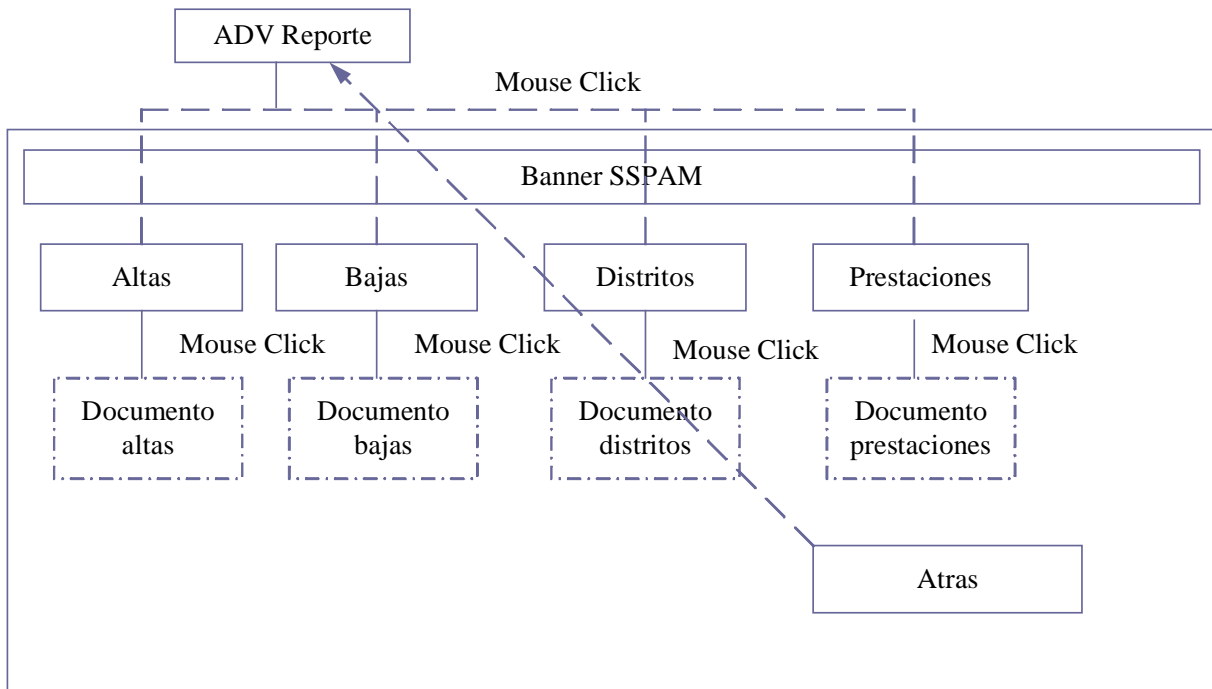
Figura 3.24 ADV Reportes Fuente: Elaboración Propia
