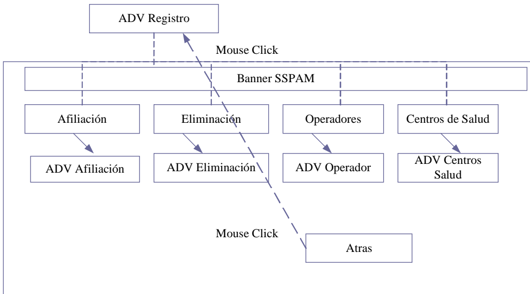
Figura 3.21 ADV Registro Fuente: Elaboración Propia
