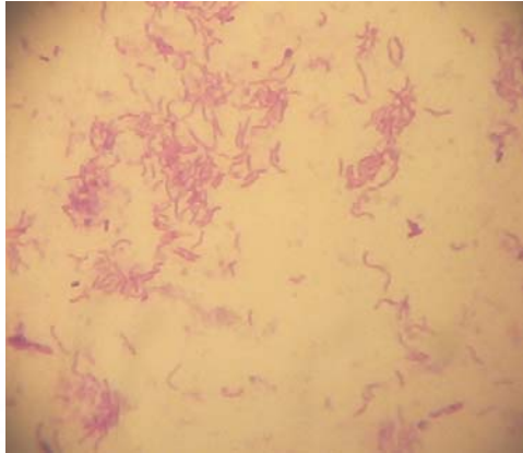
Tinción gram de Helicobacter pylori
