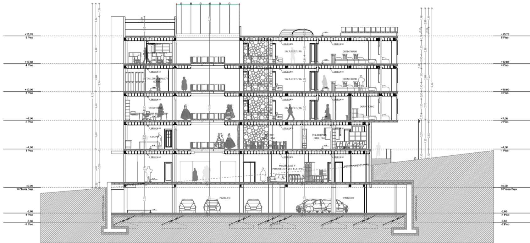
CORTE B-B
