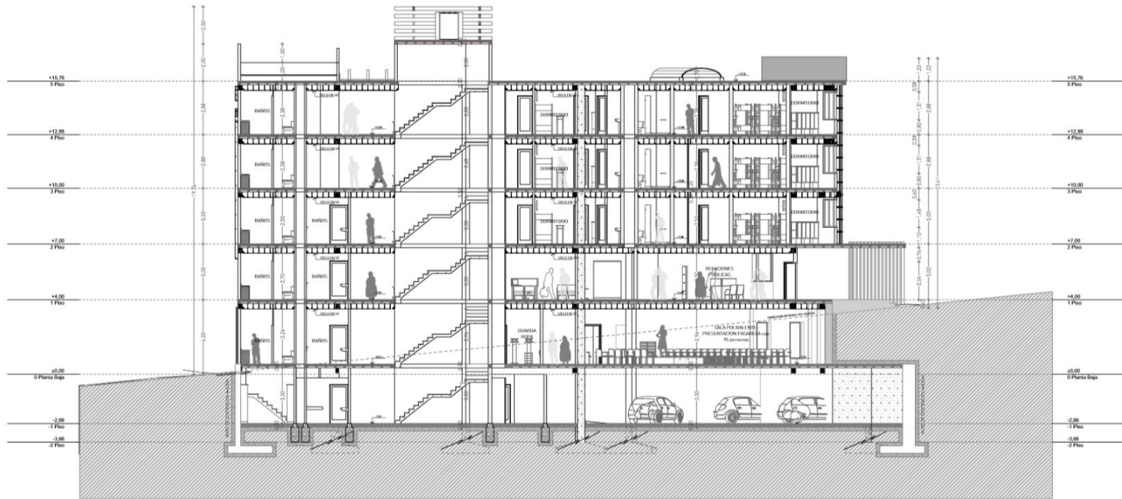
CORTE A-A
