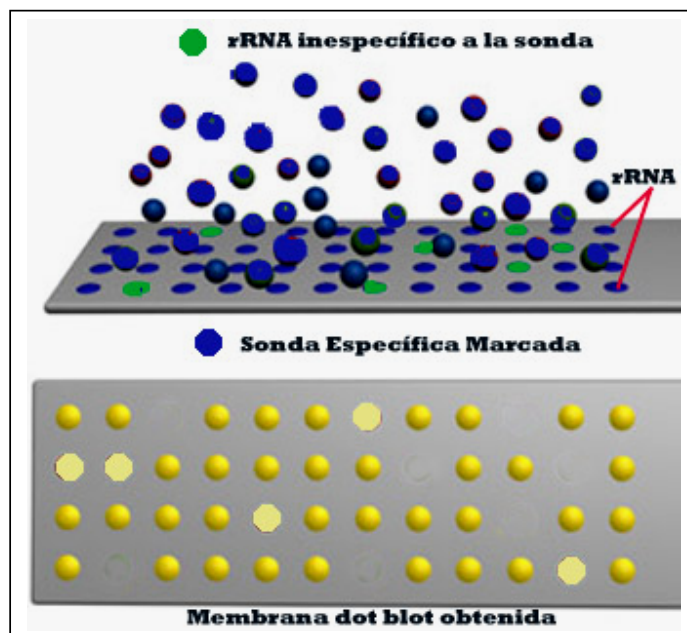
Figura 8888 . Esquema de la hibridación molecular dot blot.
