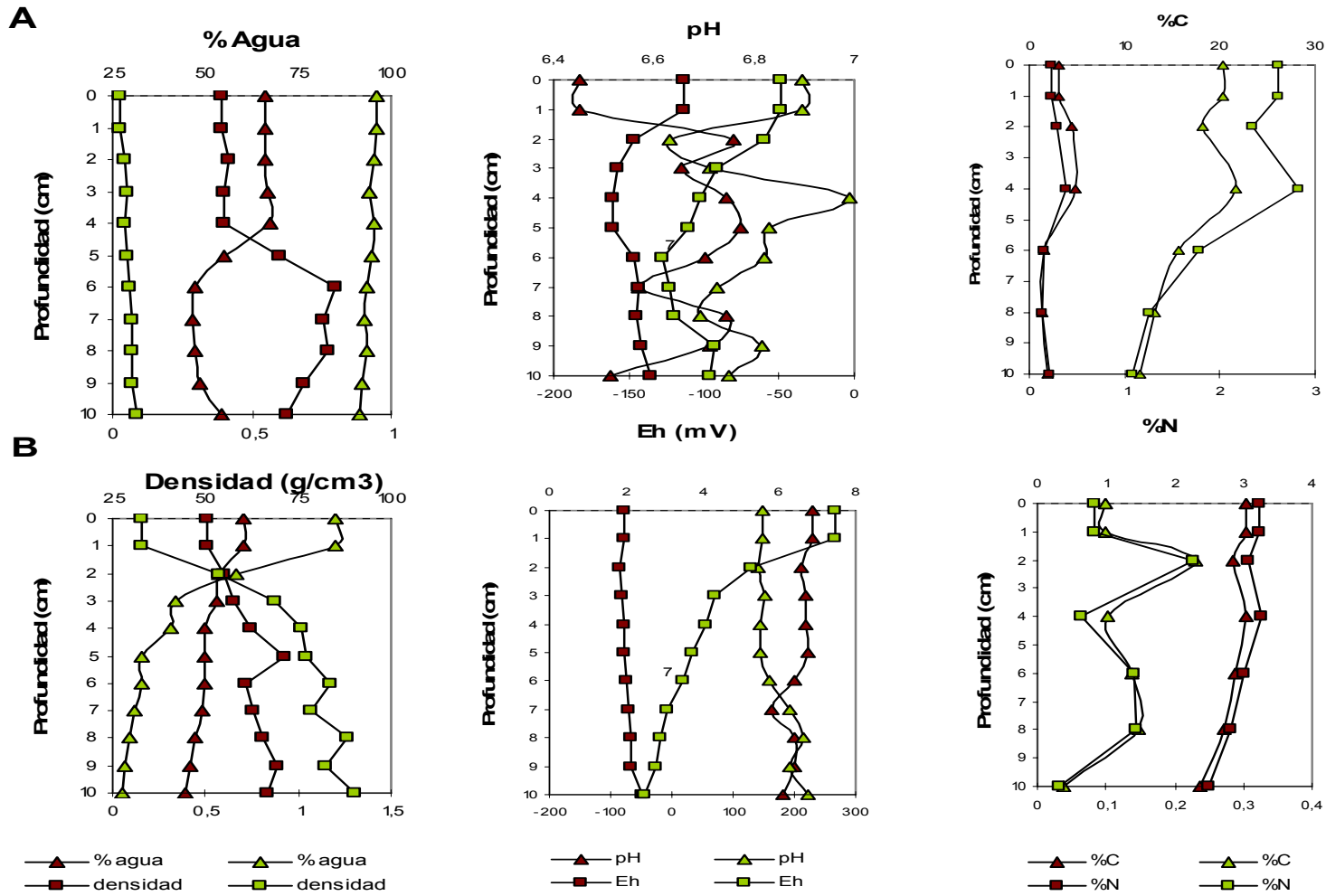
Gráfica 2222. Características fisicoquímicas y geoquímicas de los perfiles sedimentarios de Chitwara (guindo) y San Gregorio (verde)
