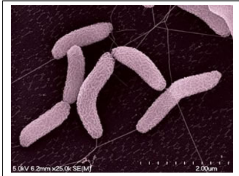
Figura 3333. Microfotografía de Desulfovibrio desulfuricans .
