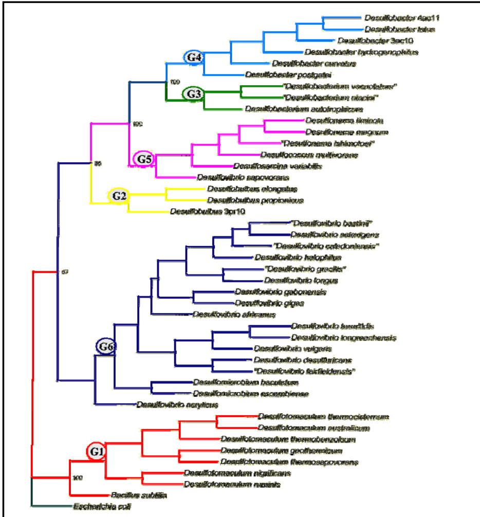
Figura 4444. Árbol filogenético basado en el 16S rRNA donde se muestran los seis linajes de bacterias sulfato reductoras (Daly et al., 2000).
