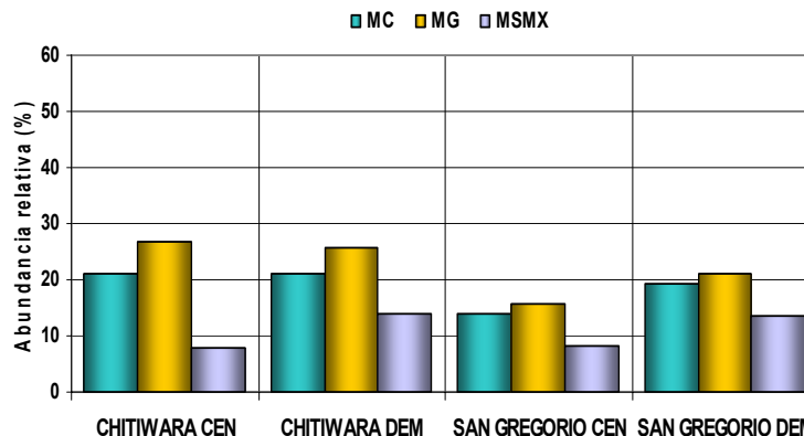
Gráfica 666. Comparación de la abundancia relativa de los sub-grupos de SRB y MA. A, Lagunas de aguas blancas; B, Lagunas de aguas negras. DFM (■), DBB (■), DSB (■), DCC (■), DSV (■), MC (■), MG (■) y MSMX (■).
