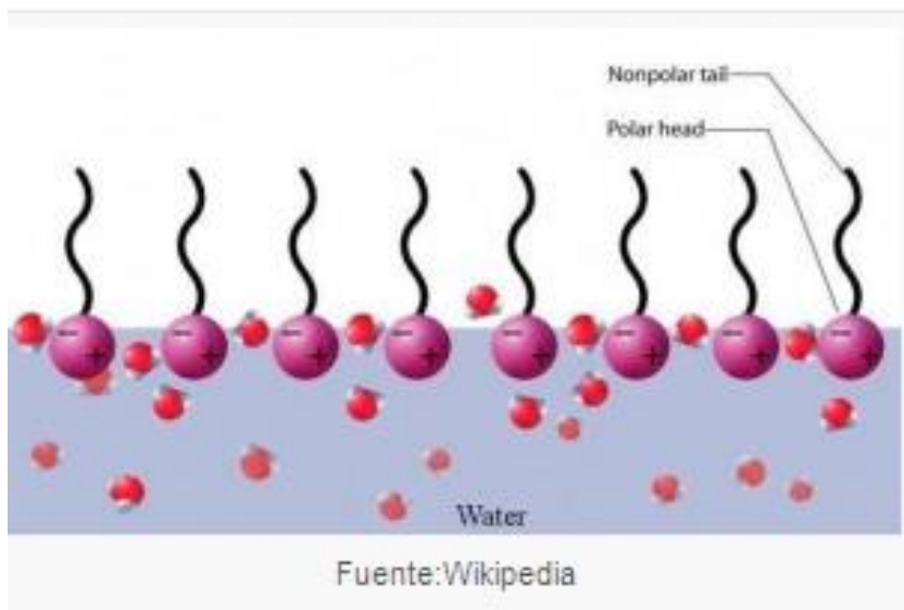
Figura 4. Distribución de las moléculas de tensoactivo (16).
