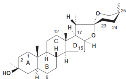
Figura 2. Estructura del spirostan. Fuente (15)
