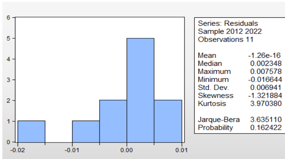
Figura 17: Test de Normalidad Residuos del Modelo
