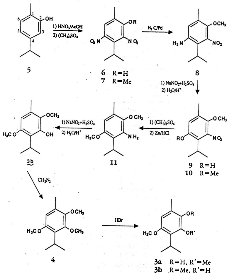
SCHÉMA 1. Synthèse de l'espintanol [3a] et de l'isoespintanol [3b].
