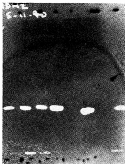
PHOTO 2. — Zymogramme pour l'enzyme IDH d'un couple de Triatoma infestans et de ses descendants (en négatif).
