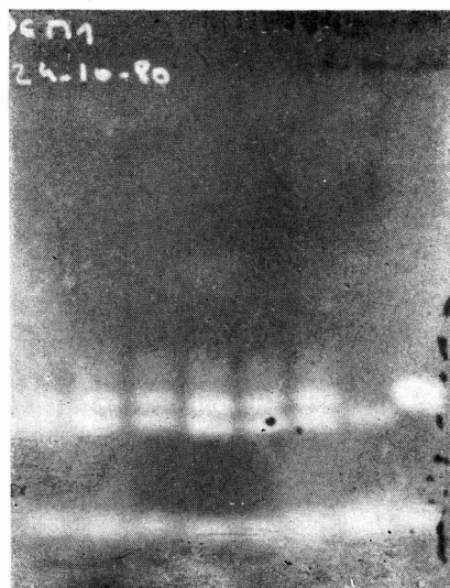
PHOTO 1. — Zymogramme pour l'enzyme PGM d'un couple de Triatoma infestans , et de ses descendants (en négatif).
