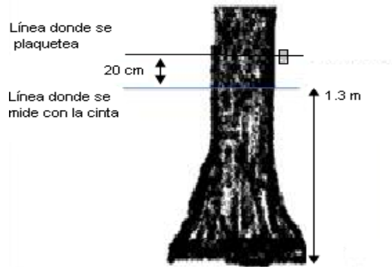
Figura 6. Forma de plaquetear por encima del diámetro medido.
